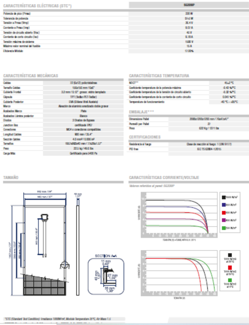
Figura 21. Características del Modelo SG330P
