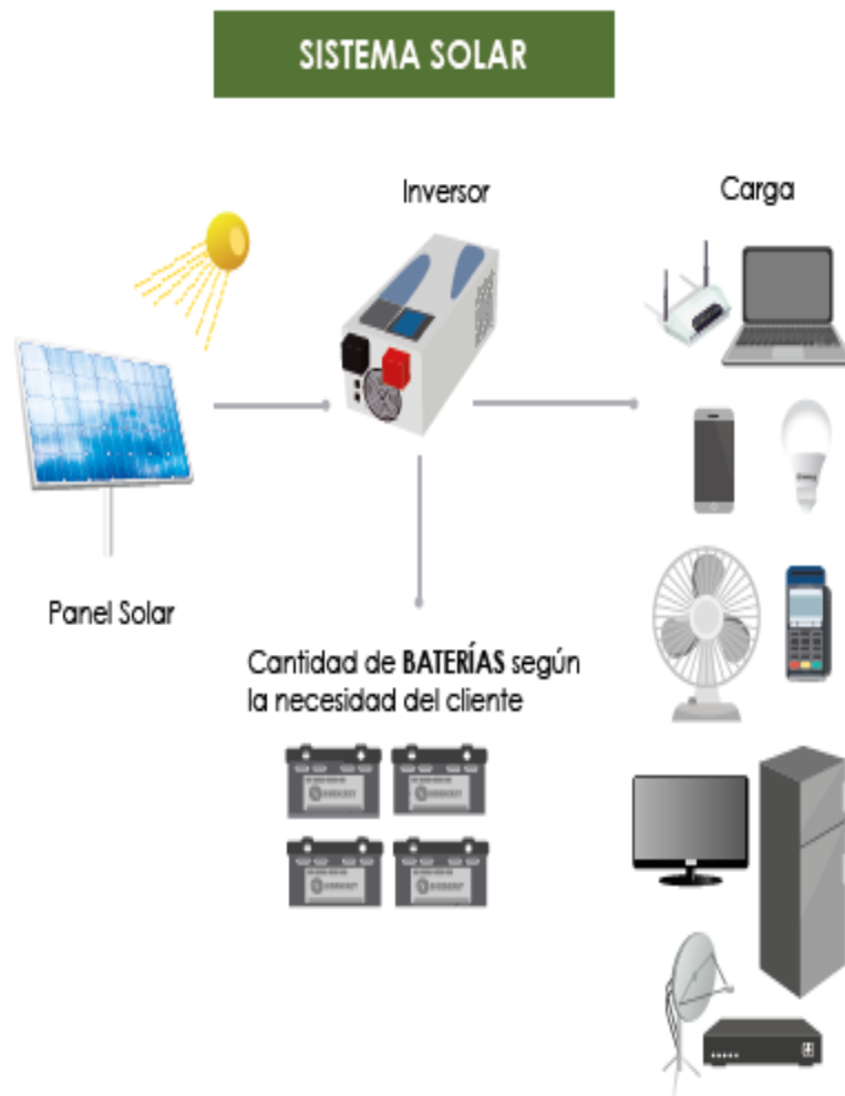
Figura 22. Sistema solar promovido por la empresa SAGET
