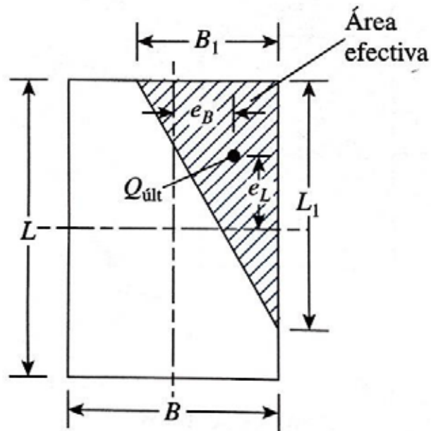
Figura 8. Área efectiva para el caso: — - - - -
