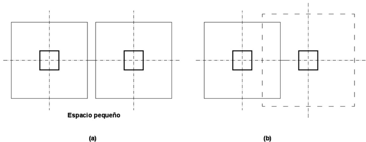
Figura 15. A.Zapatas aisladas. B.Zapatas traslapadas
