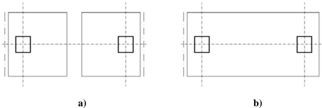
Figura 14. a) Zapatas aisladas b) Zapata corrida
