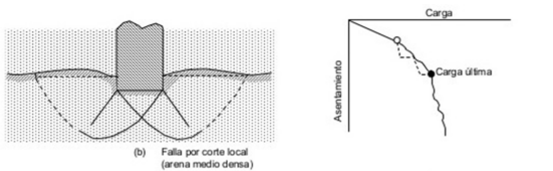
Figura 2: Falla local por corte.
