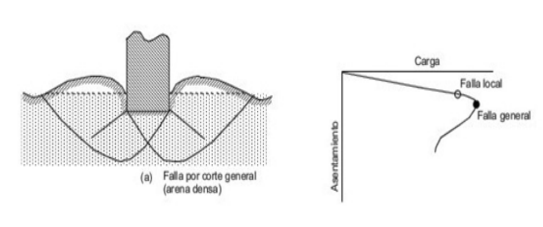
Figura 1: Falla General por corte.
