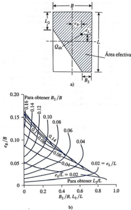
Figura 11. Área efectiva para el caso: — - — -
