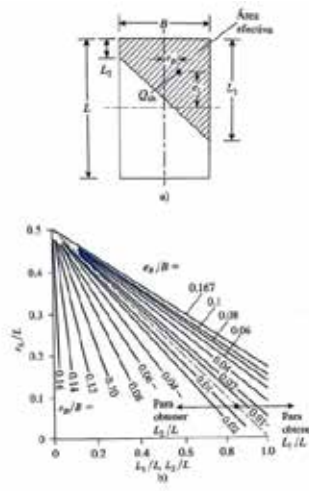
Figura 9. Área efectiva para el caso: — — —
