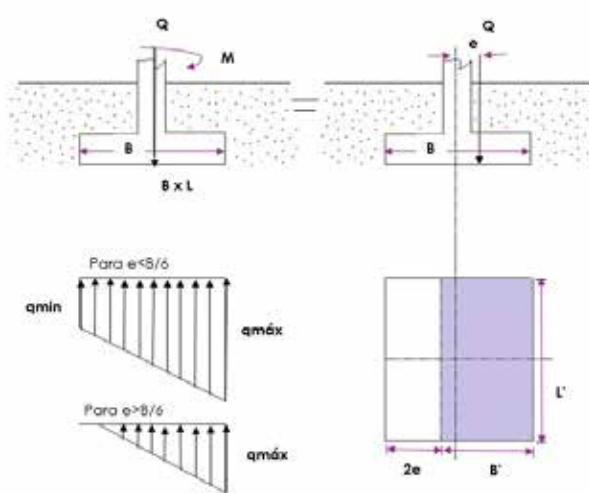
Figura 5. Cimentaciones cargadas excéntricamente Fuente: Braja Das, 1999.
