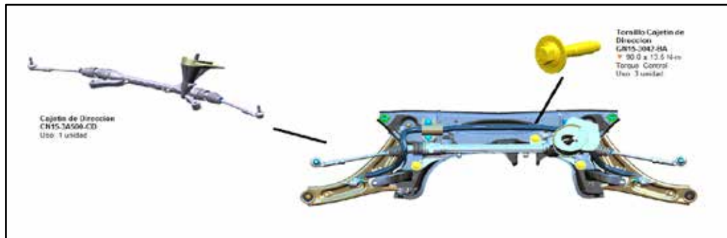
Figura 27. Subensambladura Central Sub Frame 3-3
