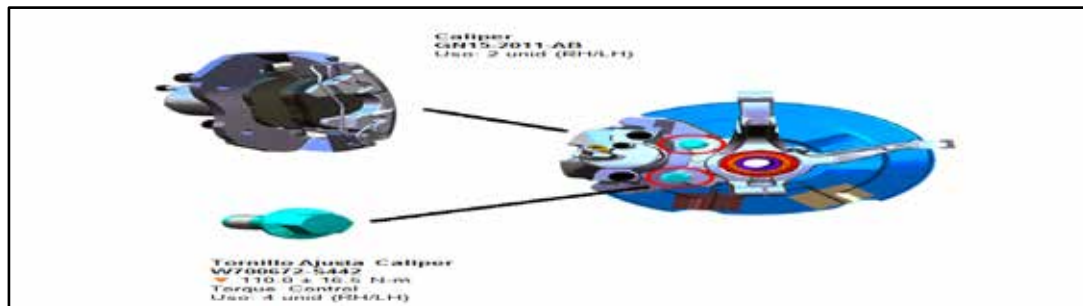
Figura 28. Subensambladura Caliper
