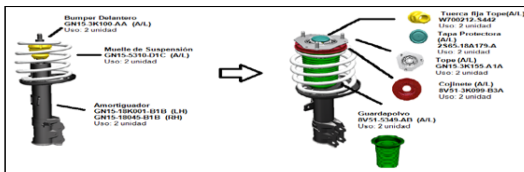
Figura 30. Subensamblado Mc Pherson
