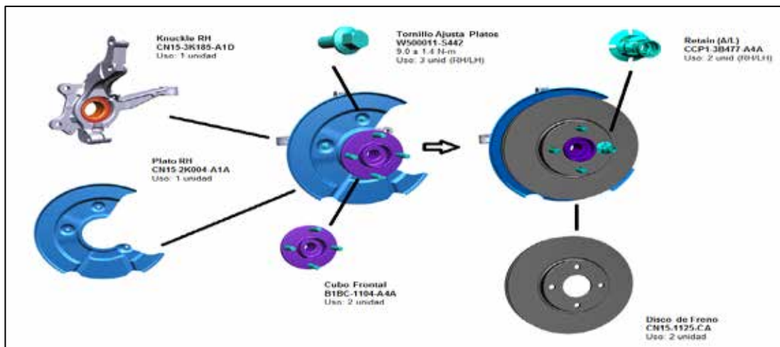
Figura 29. Subensamblado Knucle-Disco
