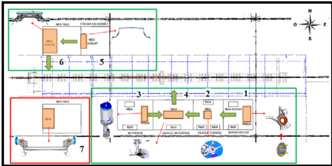
Figura 36. Diagrama de recorrido de plano propuesto para el ensamble de suspensiones
